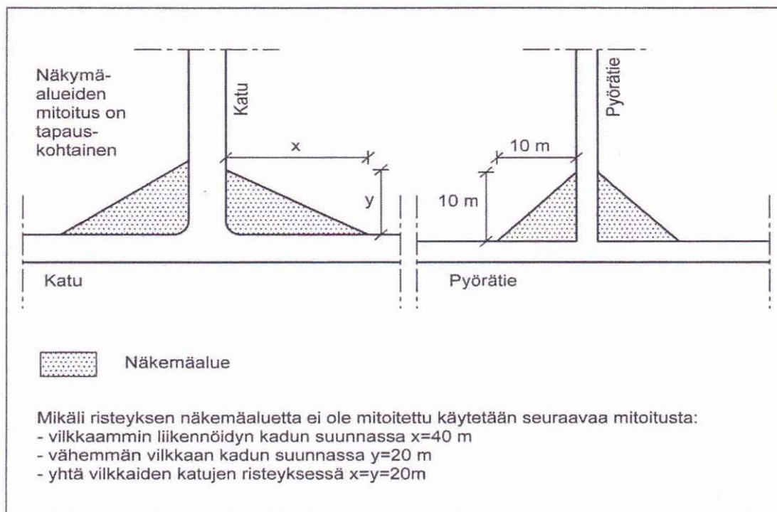
Kuva 1: Näkemäalueen mitoitus
